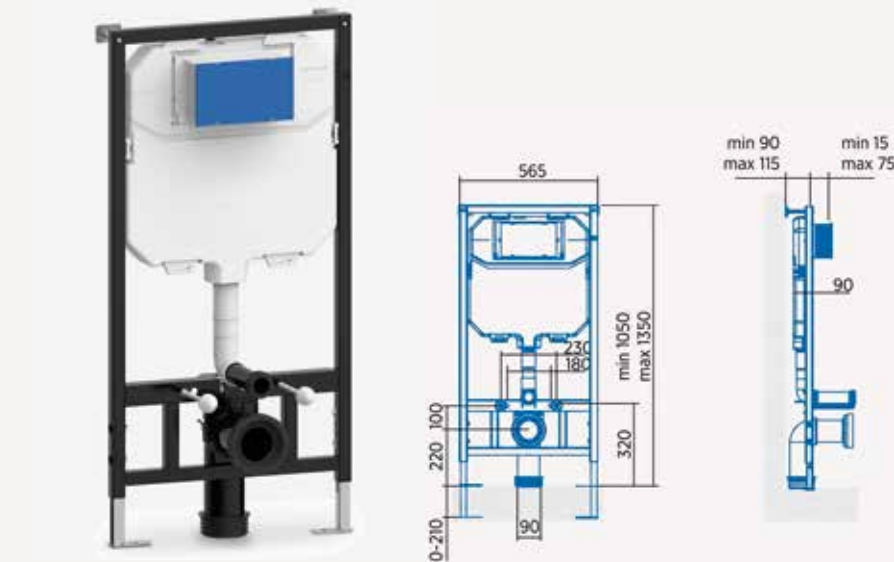
Bastidor con cisterna 1050-1350 x 56,5 cm
