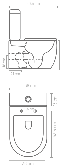
Dimensiones.
