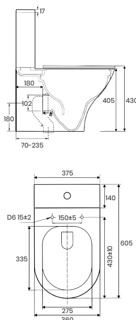
Dimensiones.
