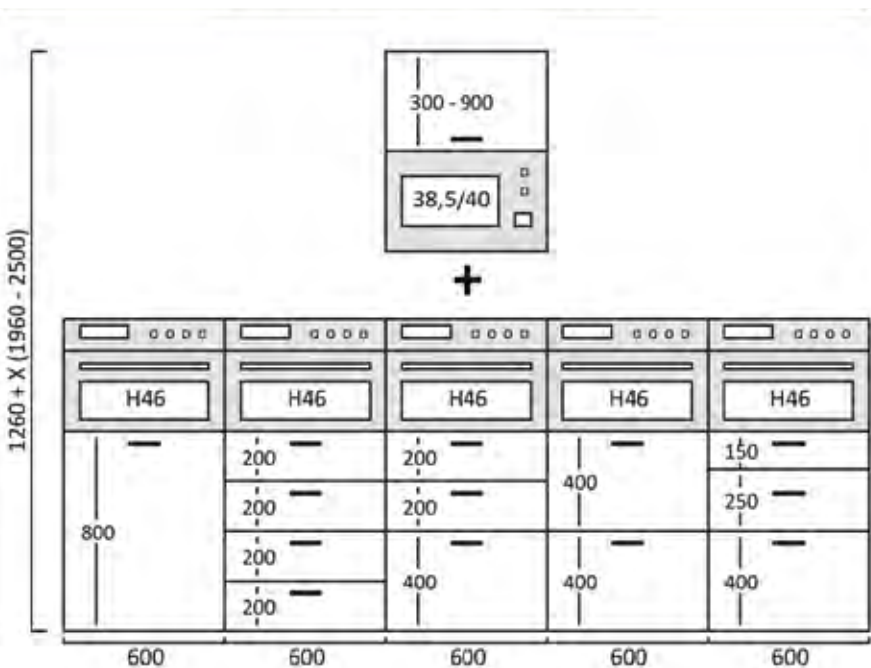
COLUMNA HORNO MICRO 1260 + X (H46)
