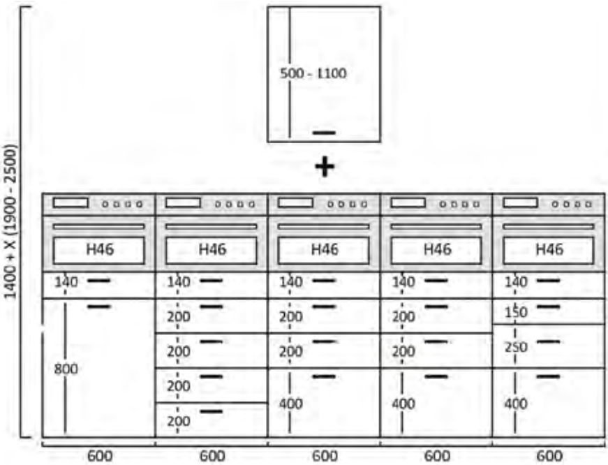
COLUMNA HORNO 1400 + X (CON CAJÓN DE 14)
