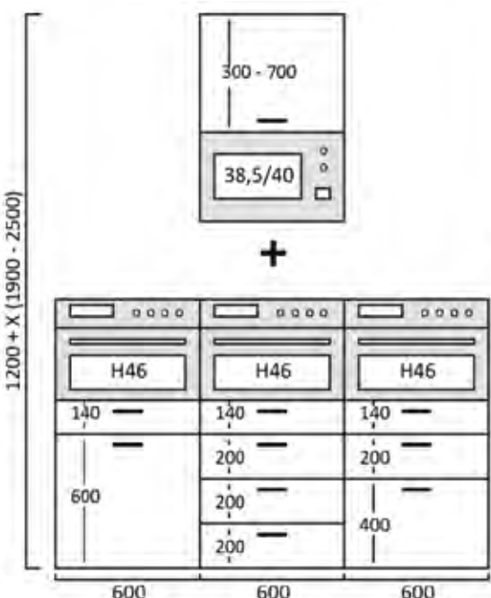
COLUMNA HORNO MICRO 1200 + X (H60)
