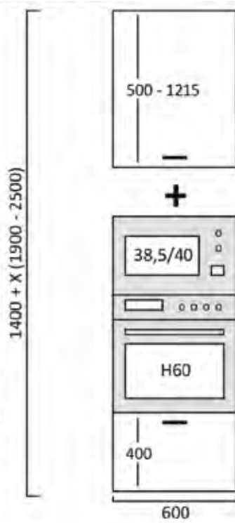
COLUMNA HM 1400 + X
