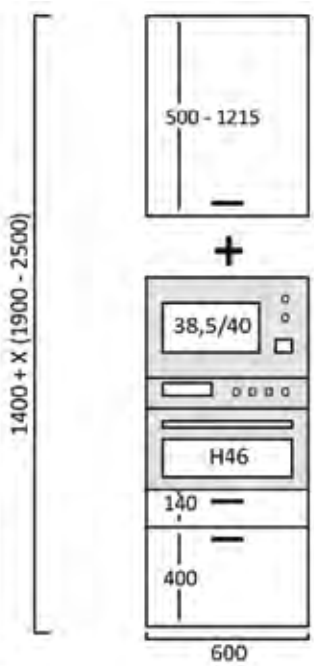
COLUMNA HM 1400 + X
