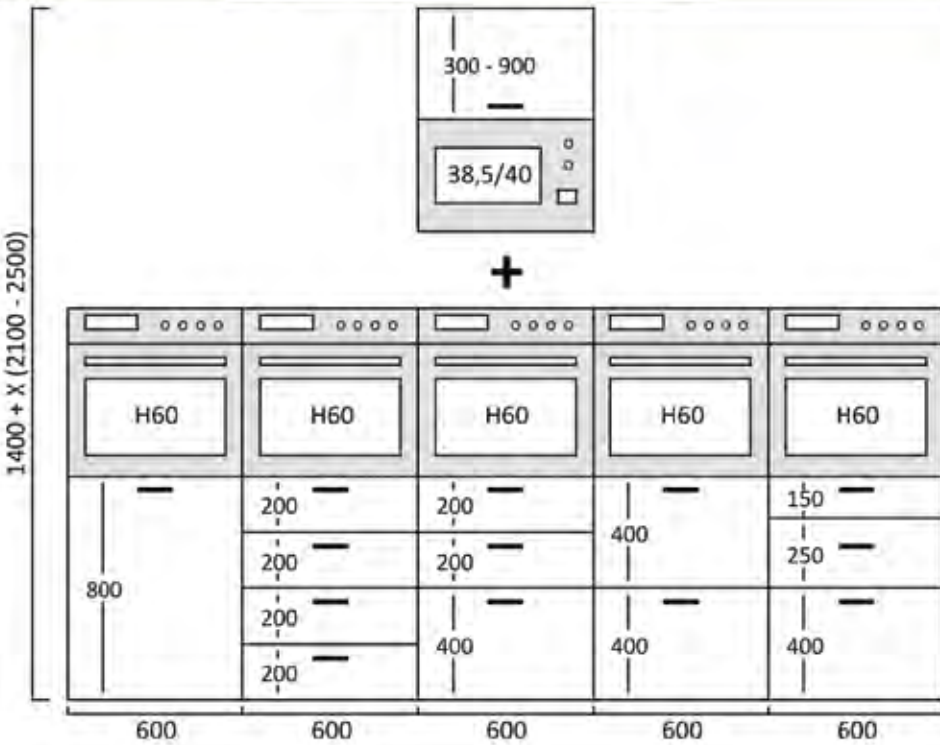
COLUMNA HORNO MICRO 1400 + X (H60)
