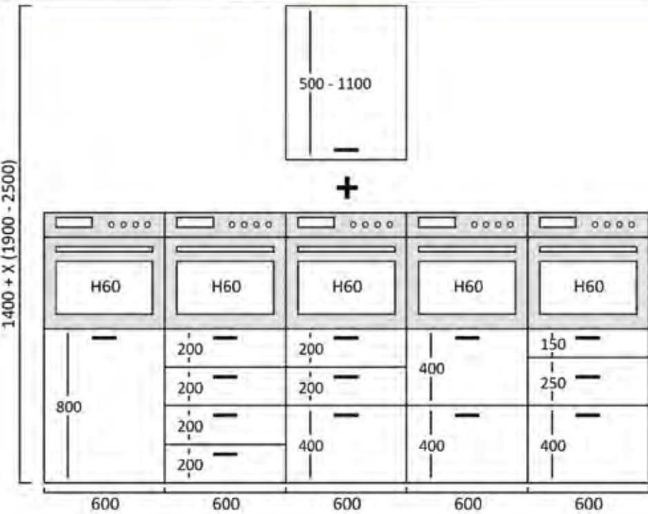
COLUMNA HORNO 140 + X
