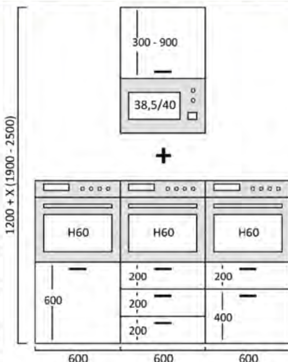
COLUMNA HORNO MICRO 1200 + X (H60)
