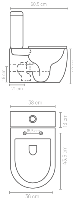
Dimensiones.
