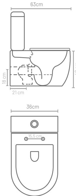
Dimensiones.
