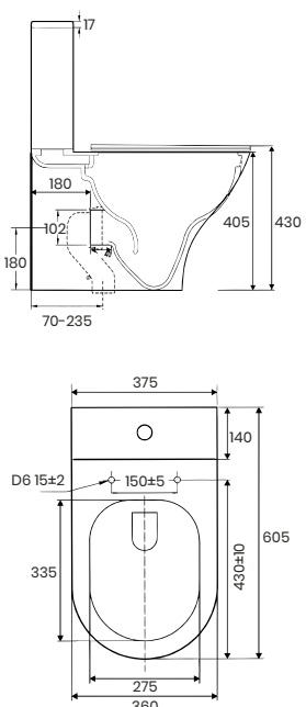
Dimensiones.
