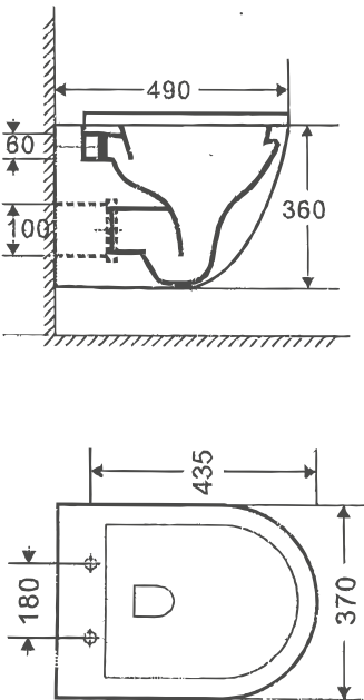
Dimensiones.
