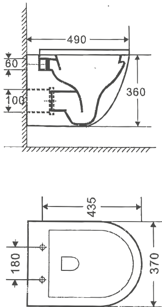
Dimensiones.
