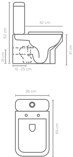
Dimensiones.
