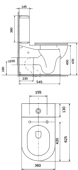
Dimensiones.
